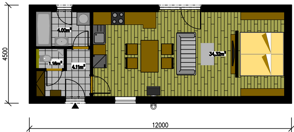
PŮDORYS 1.N.P.
