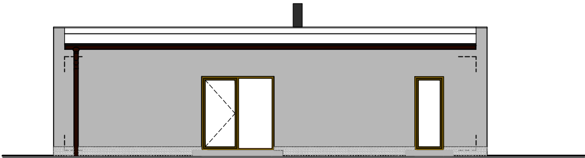
POHLED
