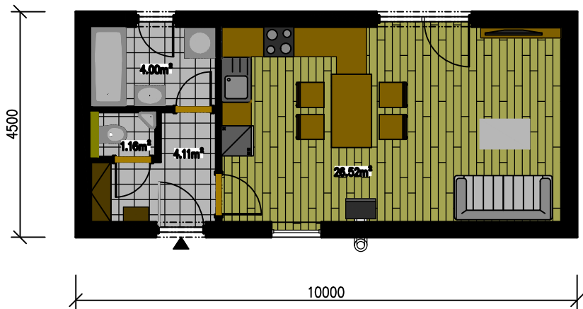
PŮDORYS 1.N.P.
