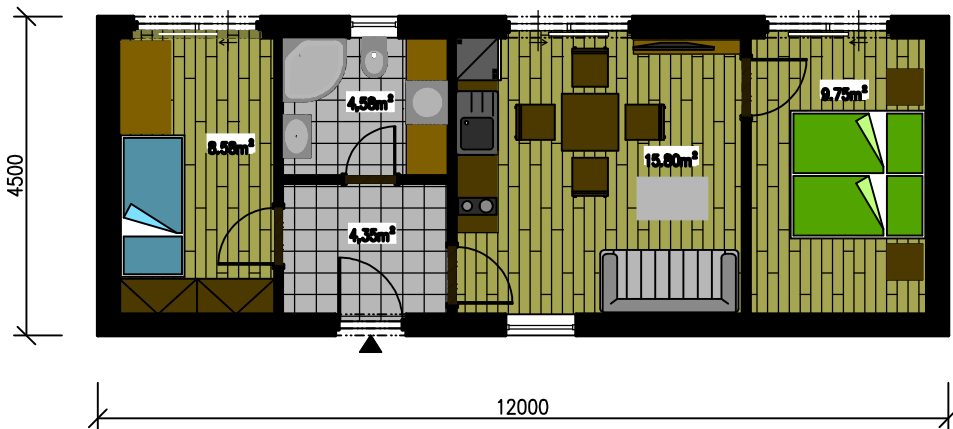
PŮDORYS 1.N.P.
